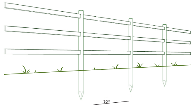
Colorado-staket med 3 slanor
